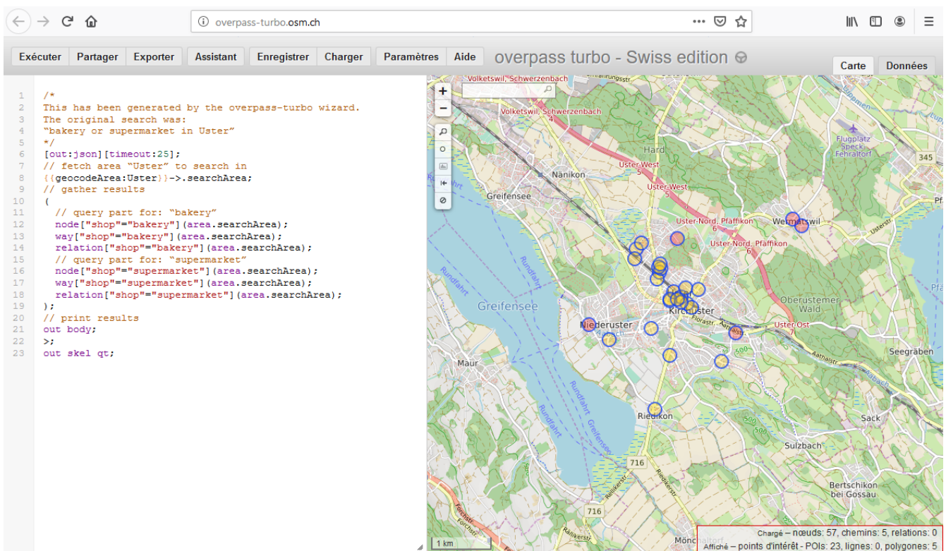
Illustration 3. Résultat de la requête de l'assistant
